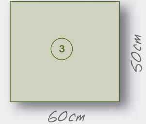
Seitenwände (2x)
